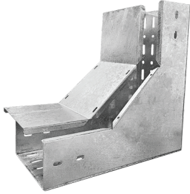
VERTICAL INSIDE 90° โค้งขึ้น (เปิดใน)
