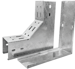
VERTICAL OUTSIDE 90° โค้งขึ้น (เปิดนอก)
